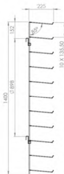
GALERIE 11 BROCHES 6153028
